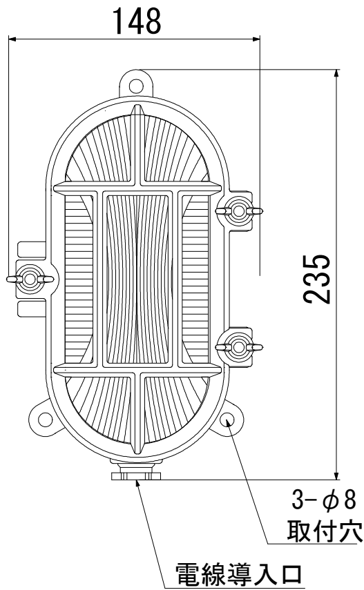
《《取付面 寸法図》》
