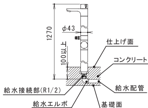
参考施工図(mm)
