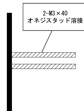
(側面図)
