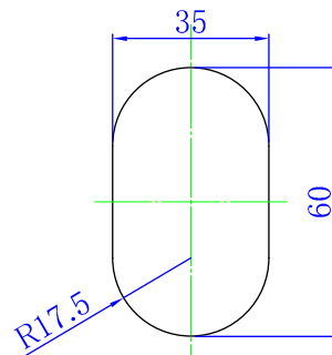
配線穴詳細図 (1/2)
